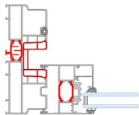
Vleugel buiten - Ouvrant ext. - Vent outside
